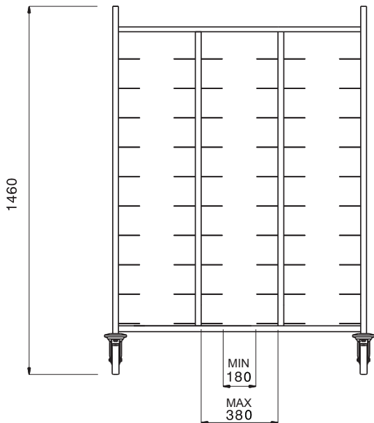
Alzado
